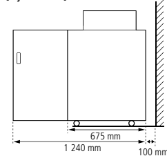
[zij aanzicht]
